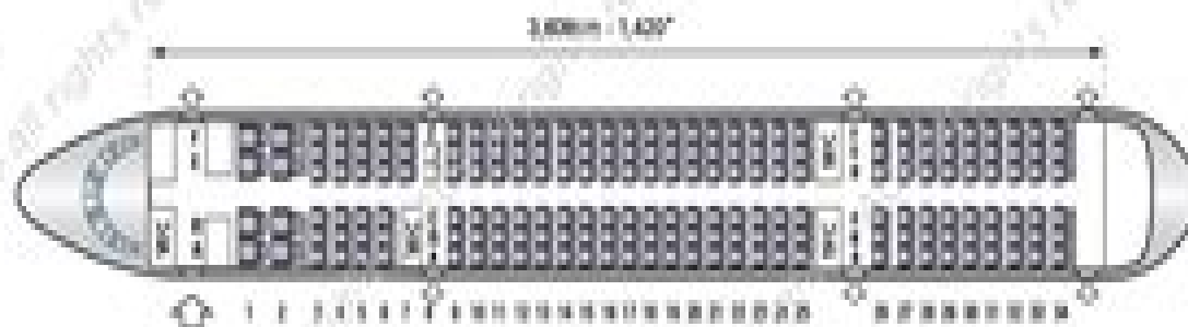
Boeing B757-200
