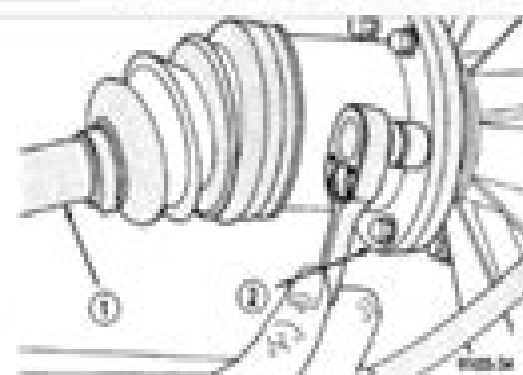
Fig. 2 Pernos internos del semieje
