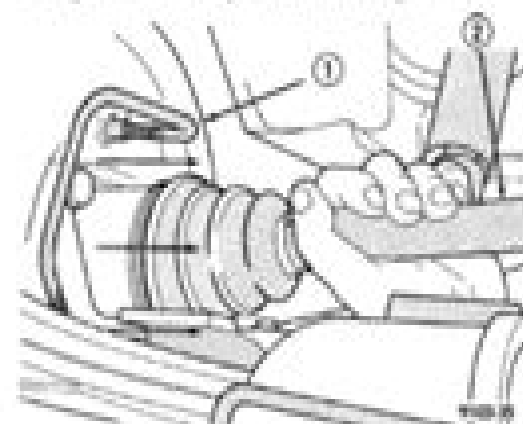
Fig. 3 Desmontaje del semieje
