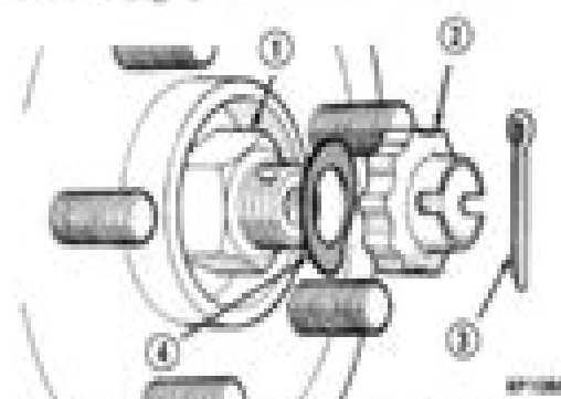
Fig. 1 Pasador, contratuercas y arandela de muelle
