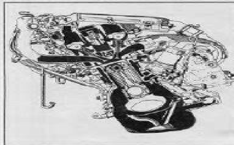
Двигатель 3S-GTE.
