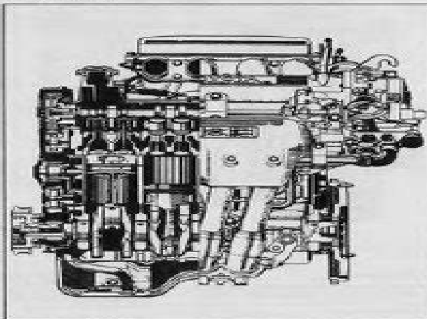
Двигатель 3S-GE.
