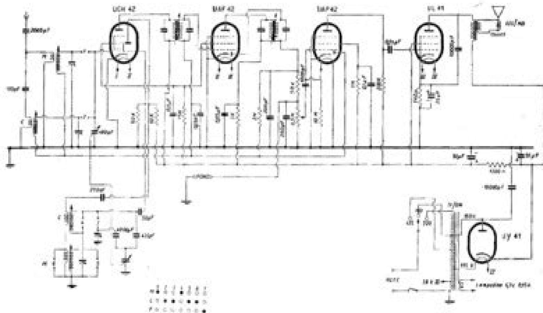
PERA RADIO (Portugal) - Mod. C/12 B. Gamma d'onda in metri: M 190200 e C 11-25. Media frequenza 487 kc/s. Potenza di uscita 1 watt. Consumo 12,5 watt.
