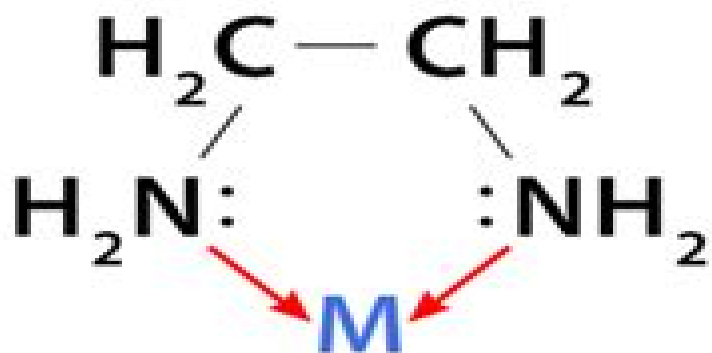
Ethylenediamine
