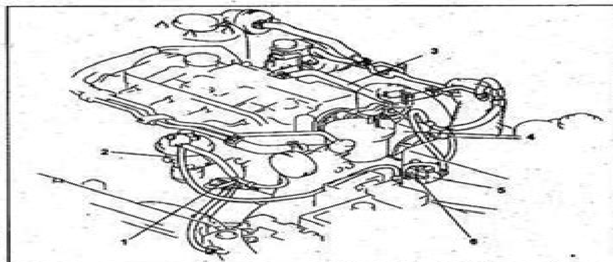
Схема расположения вакуумных линий (Mazda Capella). 1 - датчик давления наддува, 2 - электропневмоклапан системы рециркуляции отработавших газов, 3 - вентиляционный шланг, 4 - вакуумный насос, 5 - клапан №1 системы рециркуляции ОГ, 6 - клапан №2 системы рециркуляции ОГ.
