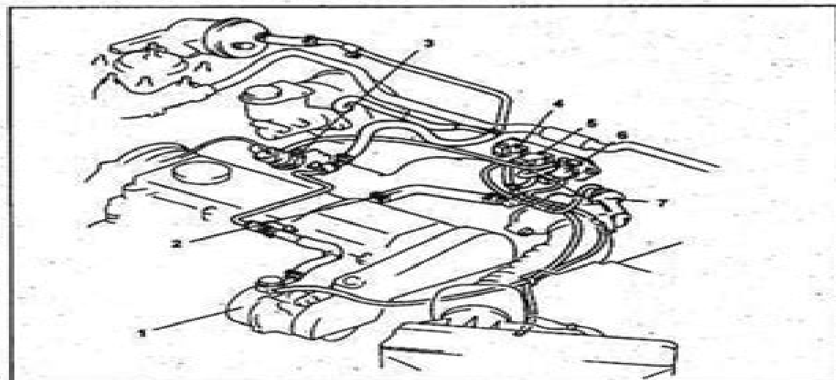
Схема расположения вакуумных линий (Mazda Familia). 1 - вакуумный насос, 2 - вентиляционный шланг, 3 - клапан системы рециркуляции ОГ, 4 - электропневмоклапан дроссельной заслонки, 5 - электропневмоклапан №1 дроссельной заслонки, 6 - электропневмоклапан №2 дроссельной заслонки, 7 - привод дроссельной заслонки.
