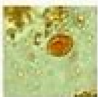
Entamoeba butschlii
