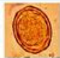
Ascaris lumbricoides
