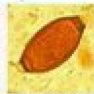
Trichostrongylus axei
