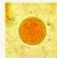
Entamoeba coli
